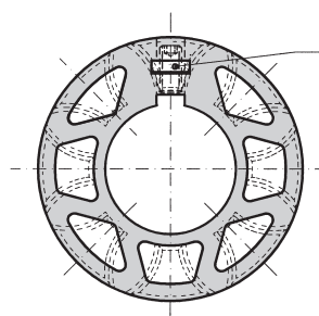
Einlegemutter
