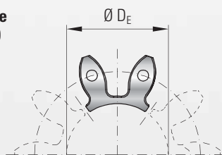
Elastomerkrans besteht aus 5x Elastomersegmenten Ausführung A / B
